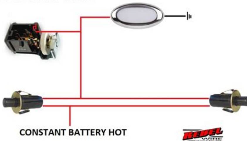
FORD DOME LIGHT WIRING
